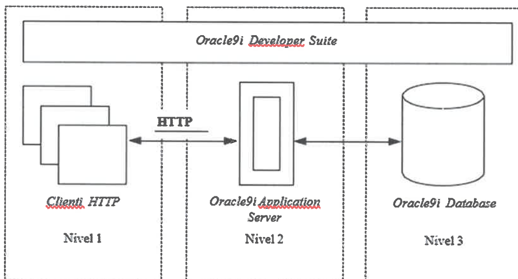
Fig. 3 Arhitectura three-tier a sistemului Oracle9i
