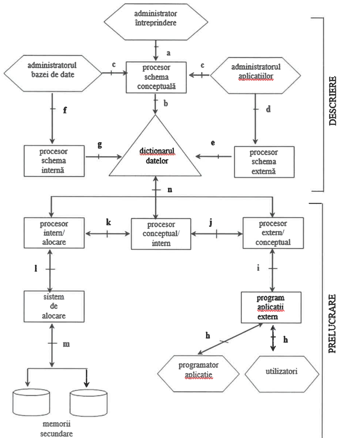
Fig. 1. Arhitectura de referință a unui SGBD.
