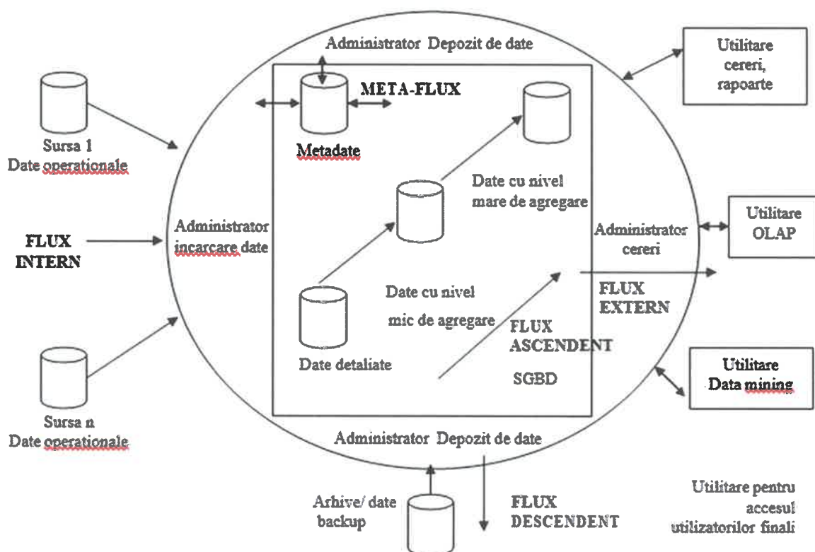
Fig 2 Arhitectura unui depozit de date
